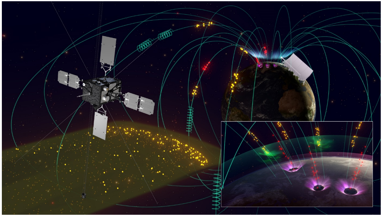
図 1: 本研究の概要 : 宇宙空間で「あらせ」衛星が「コーラス」電波とバン・アレン帯電子の観測を行い、地上では EISCAT と光学観測によって、「脈動オーロラ」と中間圏の観測を行った。
